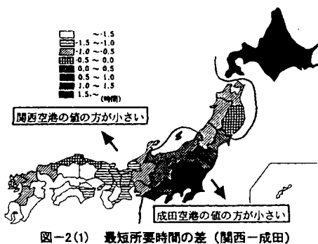
図-2(1) 最短所要時間の差(関西-成田)
