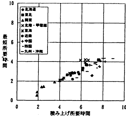
図一(1) 成田空港への最短所要時間と積み上げ所要時間
