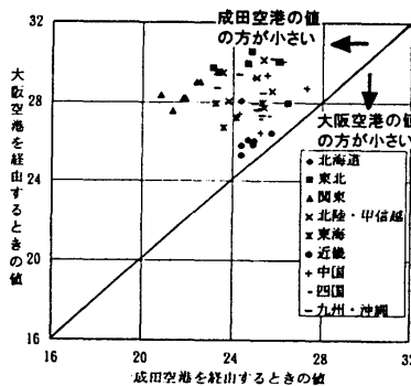
図-4(1) ロサンゼルスへの積み上げ所要時間 (1990年)
