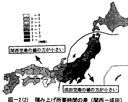
図-2(2) 積み上げ所要時間の差(関西-成田)
